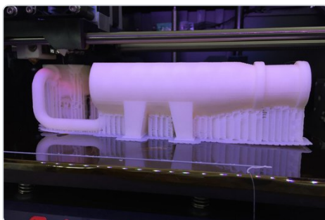
Unser 3D-Drucker im Einsatz – Behälter mit Rohrleitung
